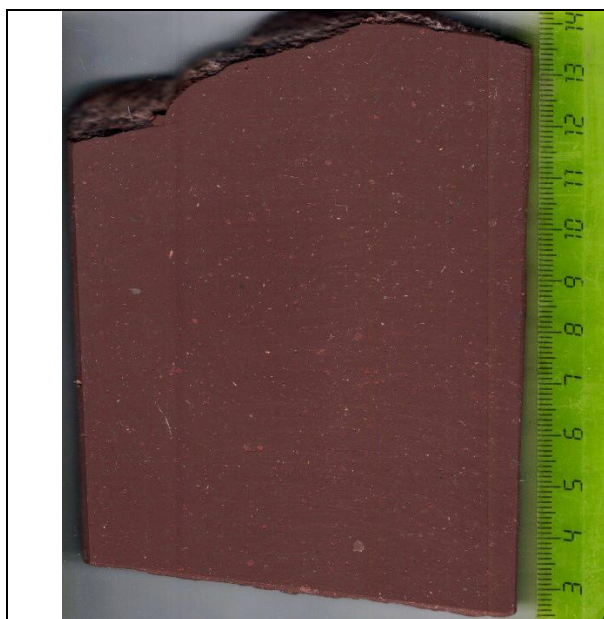
Яшмовидный боксит
